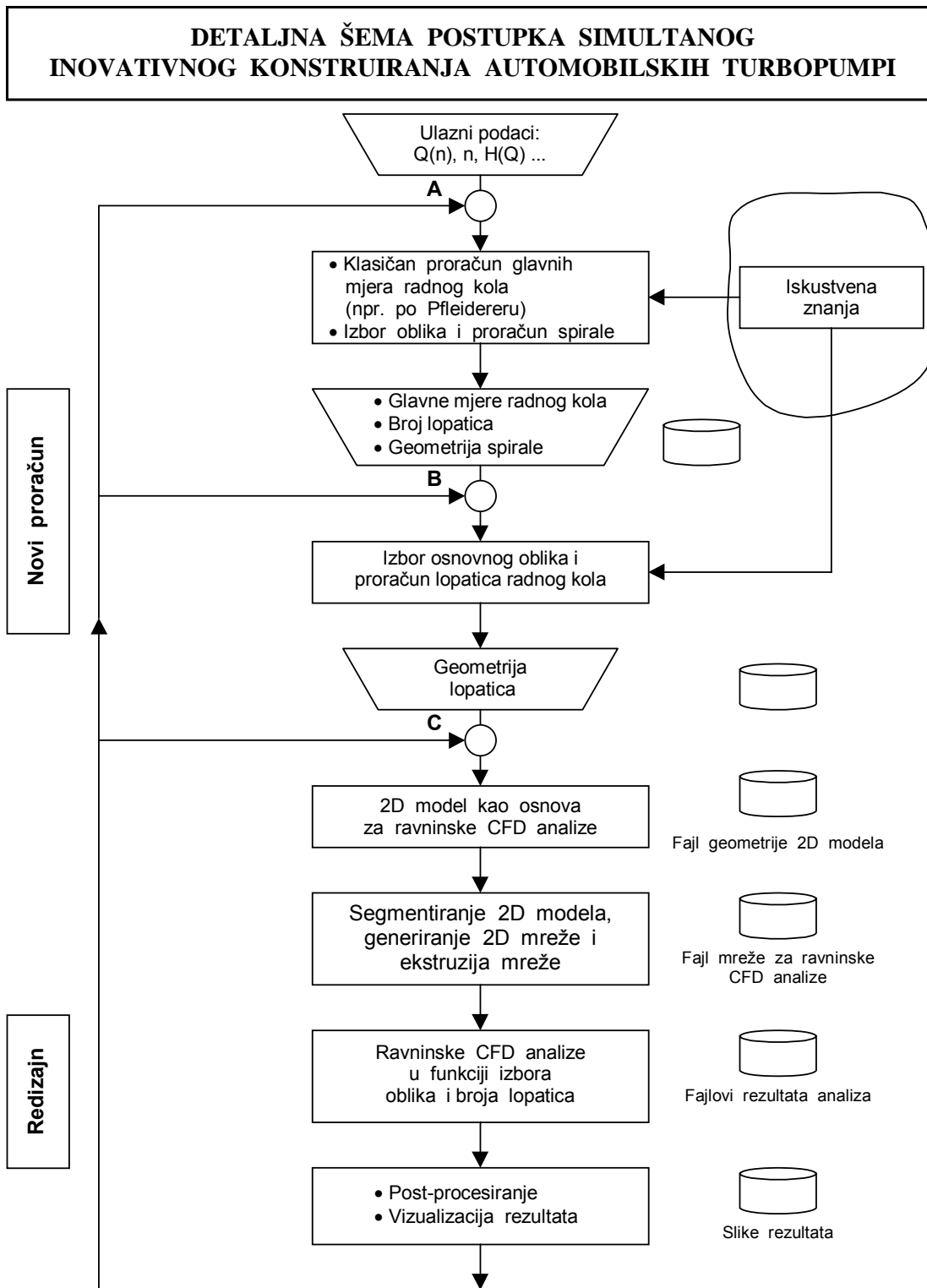
Sl. 2.4 Detaljna šema postupka simultanog inovativnog konstruiranja automobilskih turbopumpi
