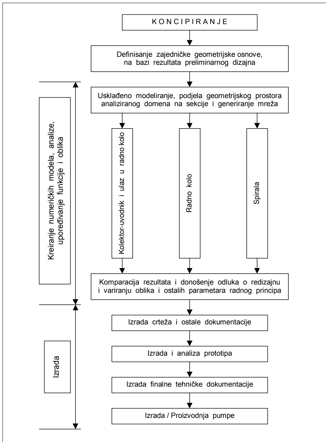
Sl. 2.3 Generalna šema postupka simultanog provođenja inovativnog konstruiranja automobilskih turbopumpi
