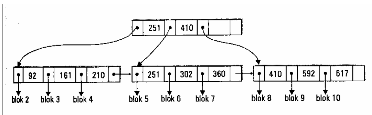
Sl. 2.4 Indeks u obliku B-stabla s dvije razine indeksa
